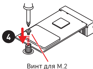
Винт для M.2
